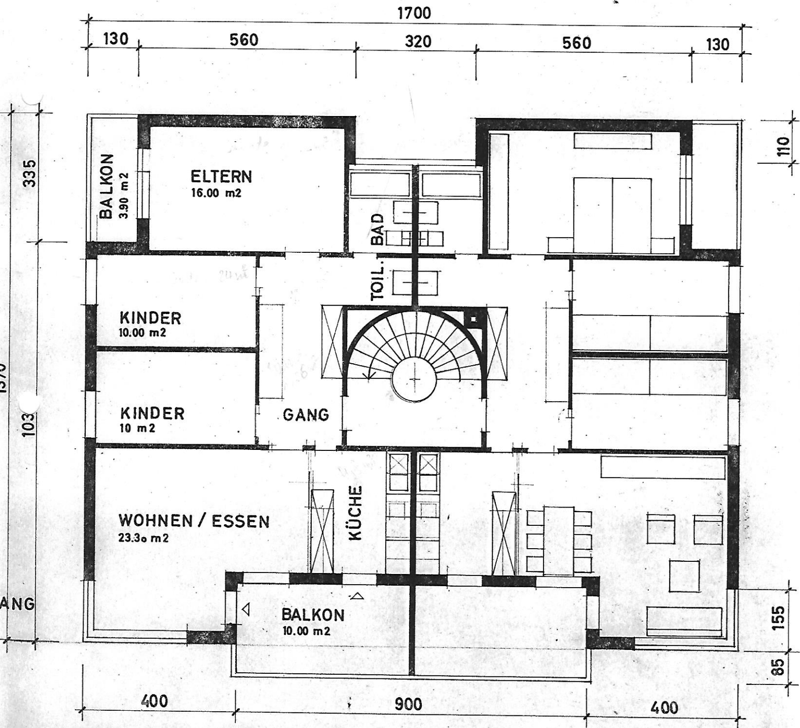
WOHNGESCHOSS
